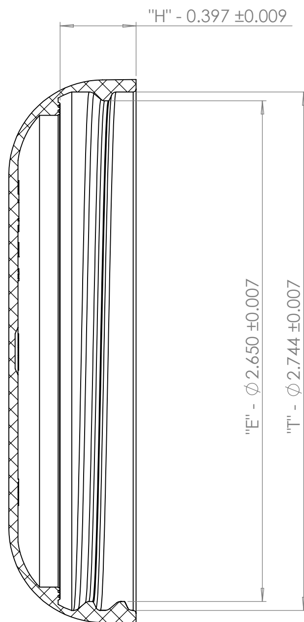
SECTION A-A
